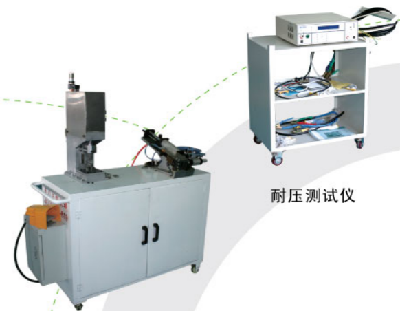
半自动电流铜头压制机 (可以自动剥皮，自动冲压)
