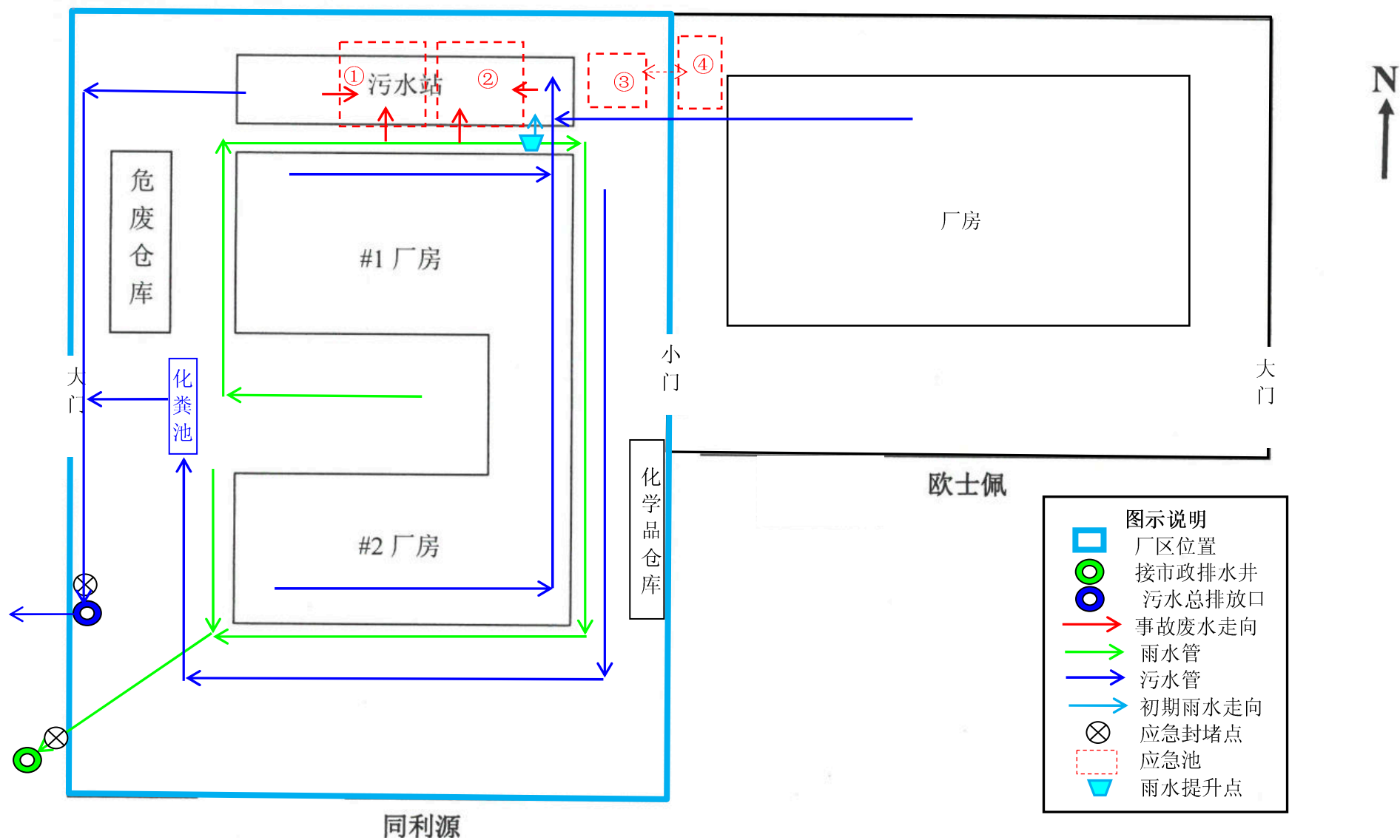
附图 5 厂区雨、污水管网示意图
