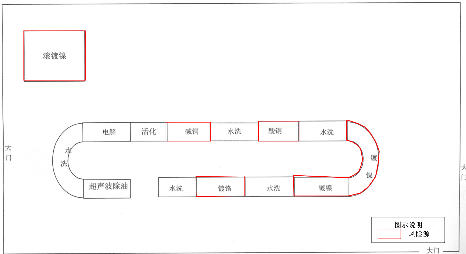
4#电镀线平面布置图
