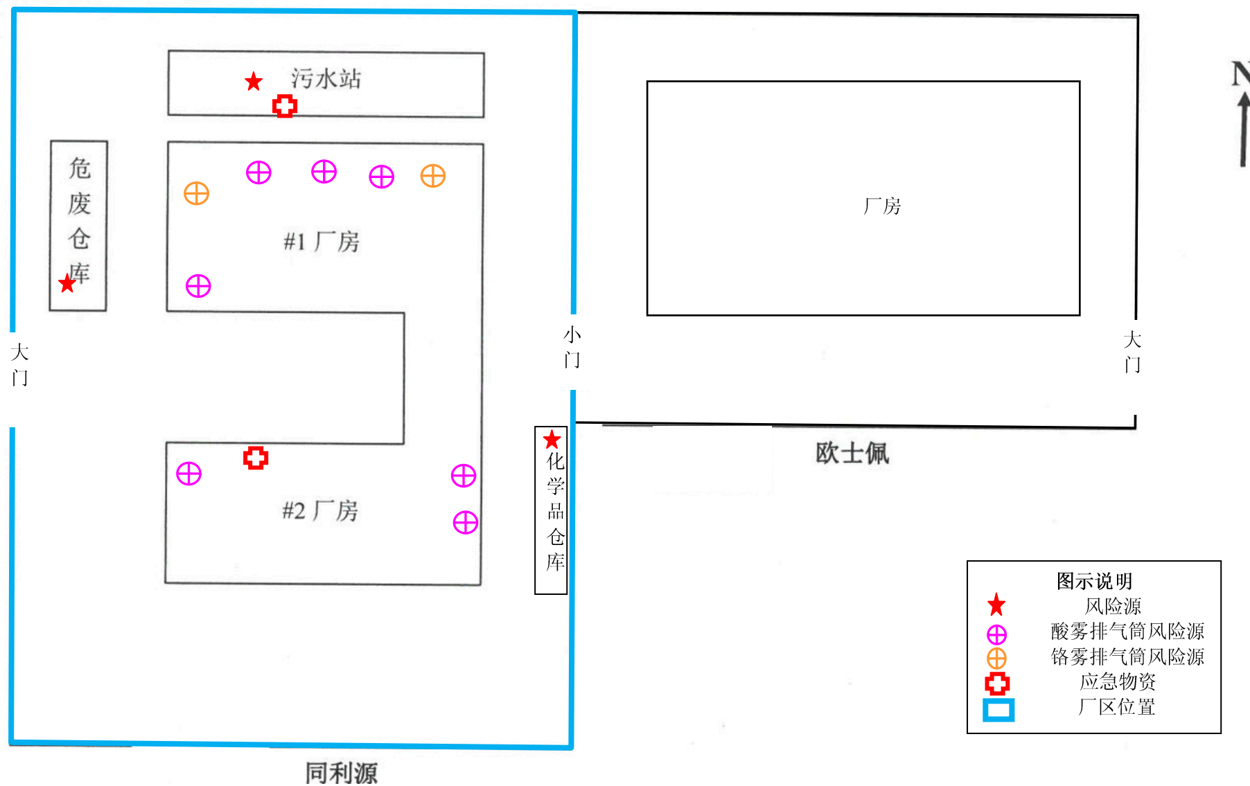
附图 6 公司及各车间平面布置图、风险源以及应急物资分布
