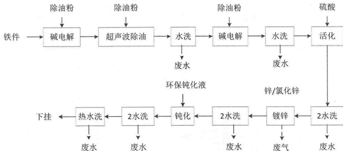
5#镀锌自动生产线工艺流程图
