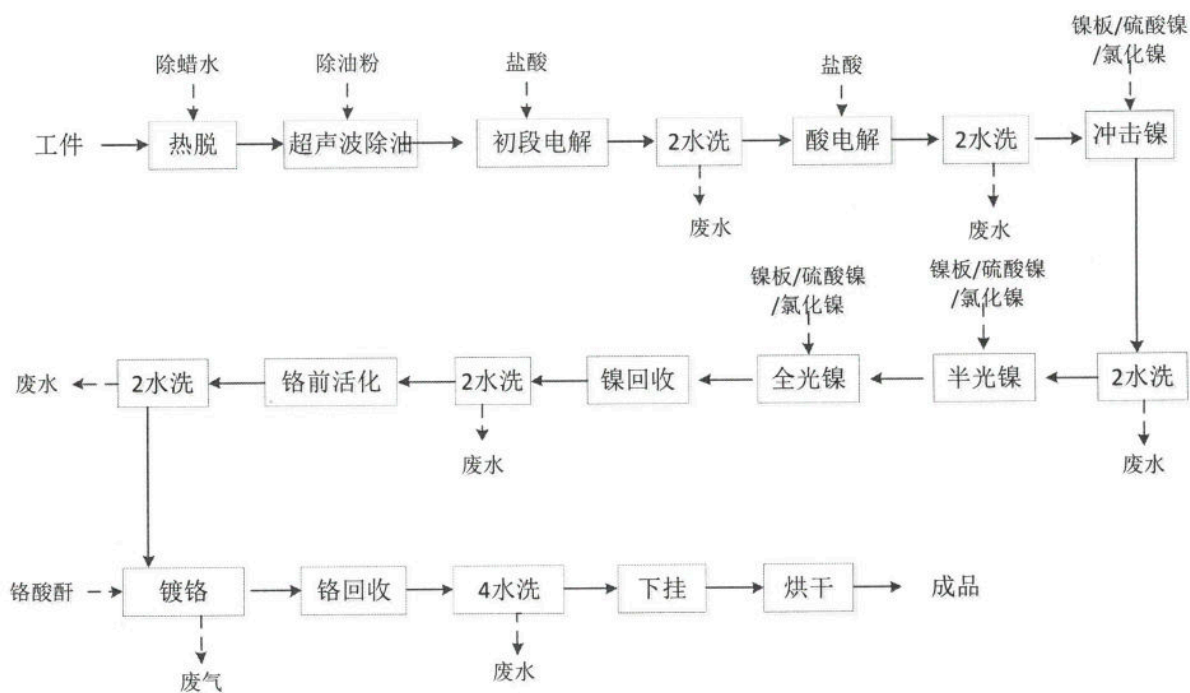
6#镍铬自动生产线工艺流程图
