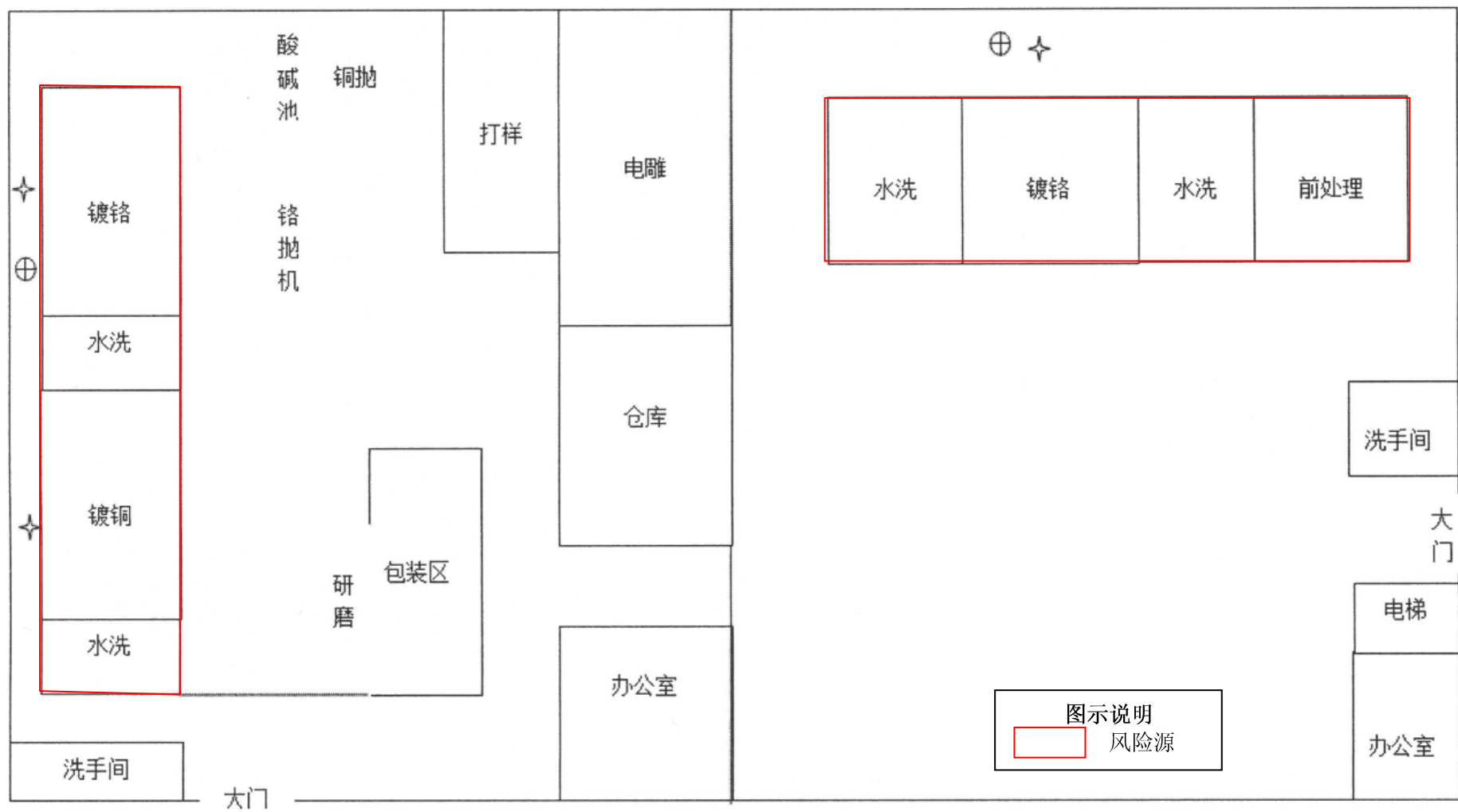
2#、3#电镀线平面布置图
