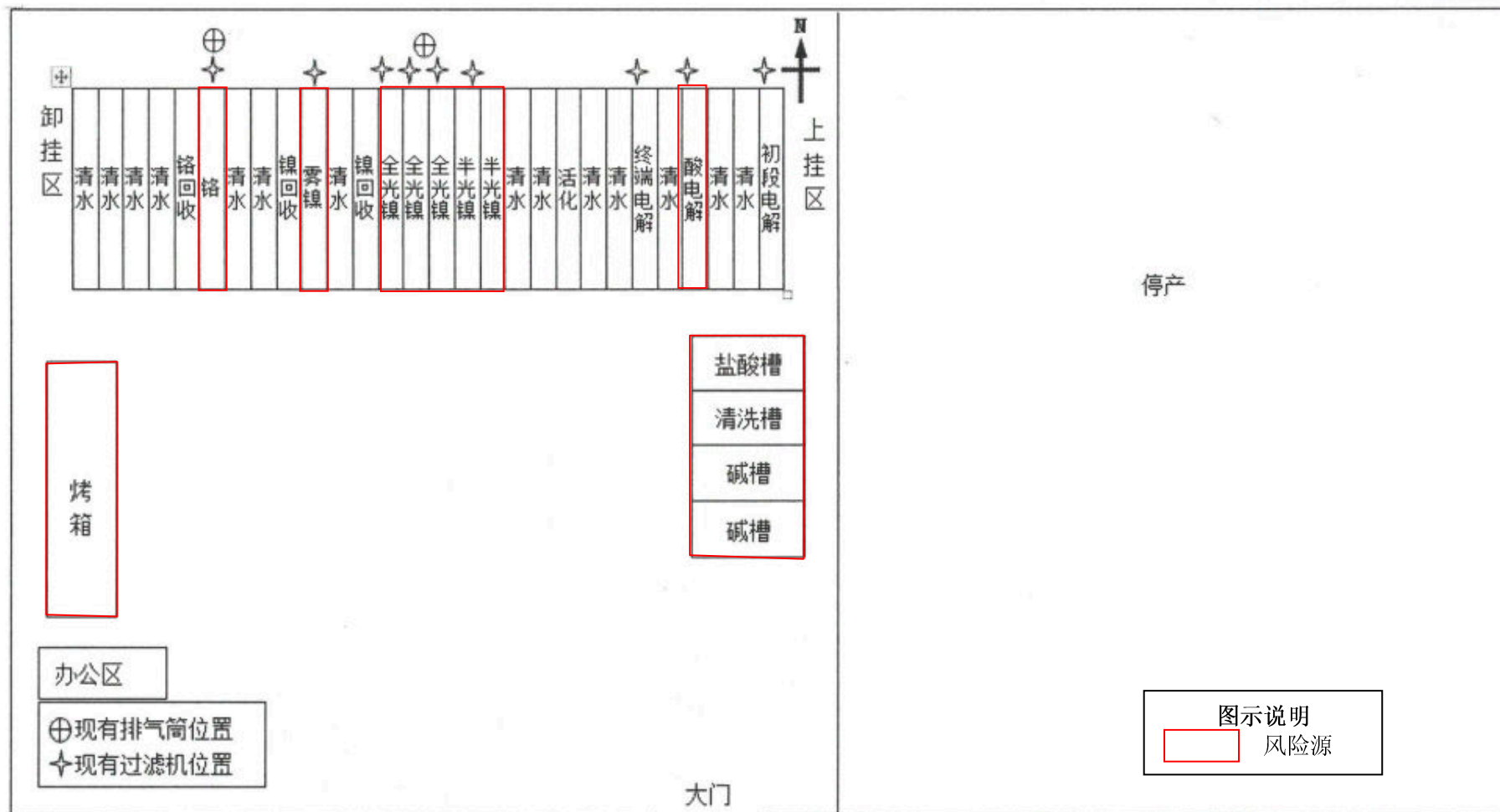
1#电镀线平面布置图
