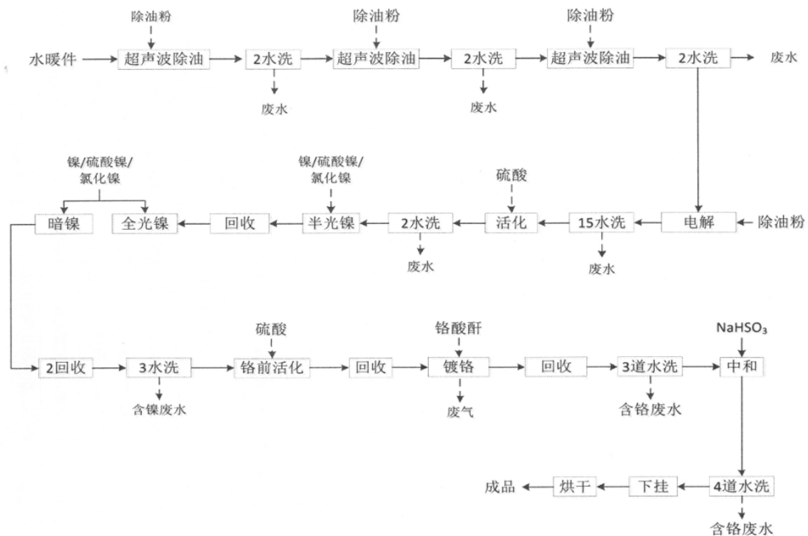
4#自动生产线工艺流程图
