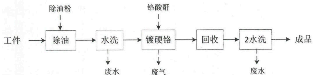
2#制版半自动生产线工艺流程图
