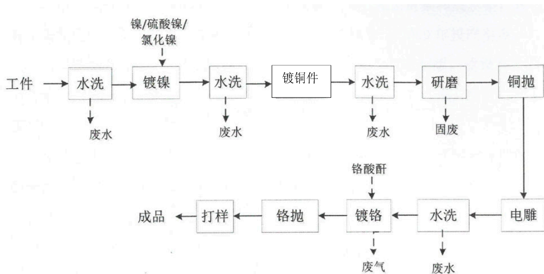
2#制版半自动生产线工艺流程图
